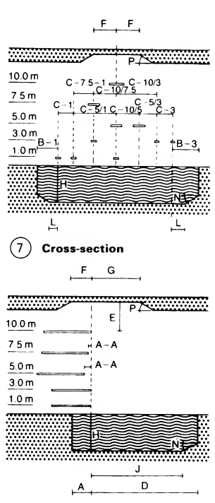
8 Longitudinal section
